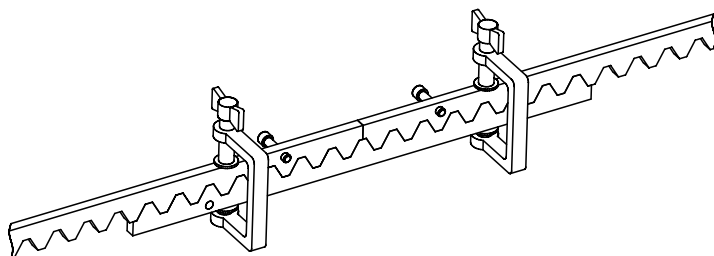
Рисунок 8. Позиционирование реек
